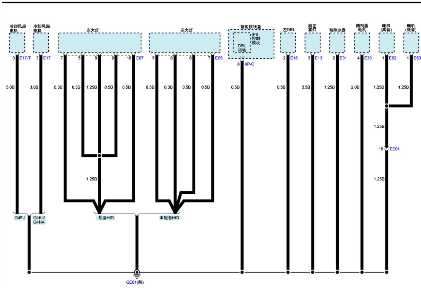
搭铁分布(5)
